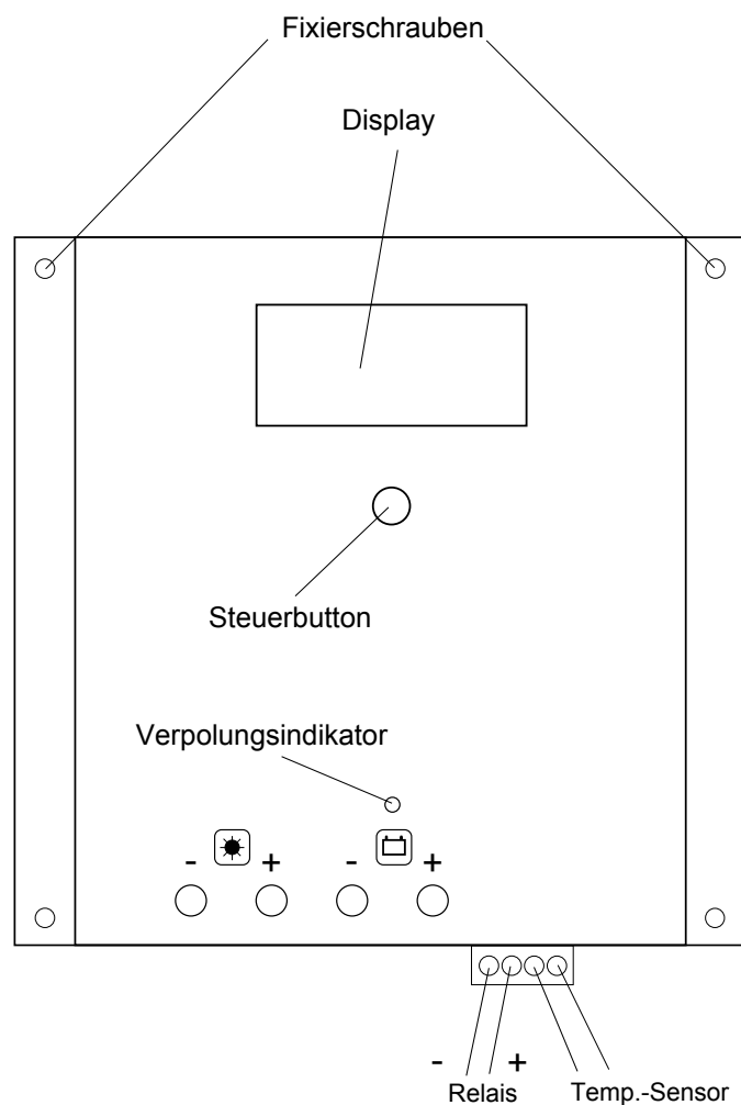
Abbildung 2: Anschlussschema
